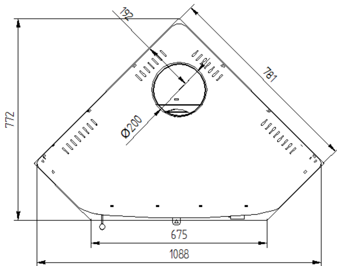
HORNO DE LEÑA MODELO HL-100 R // HL-100 RF
