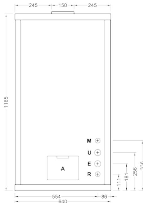
Vista posteriore (attacchi con kit)
